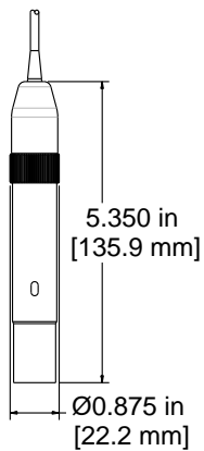
Inline Module Dimensions
