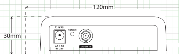
DIMENSIONS
