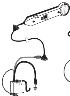
Abbildung 4a. Kabelverfolgung
