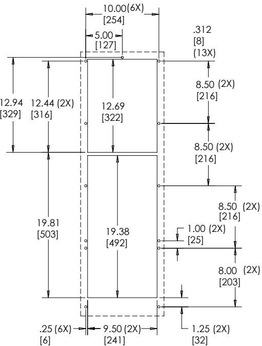
Cutout Dimensions
