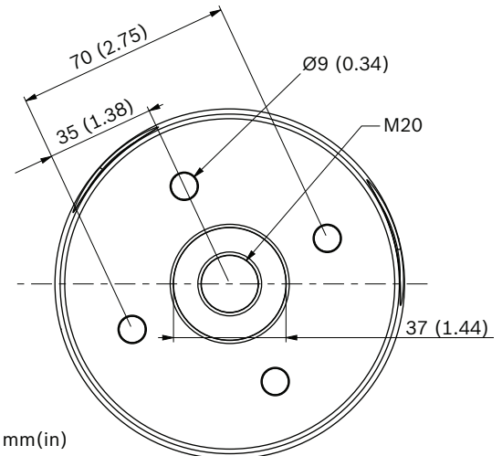
Optional pendant wall mount
