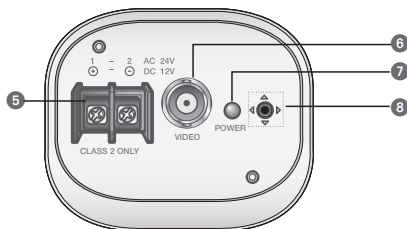
<AC24V/DC12V (SCB-2005)>
