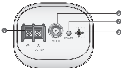
<DC12V (SCB-2005D)>
