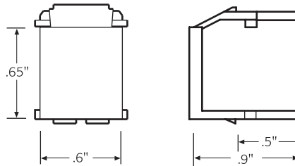
Blank Module
