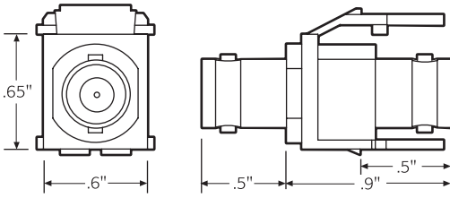
BNC Bulkhead Module
