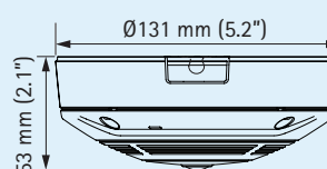
AXIS M3007-P
