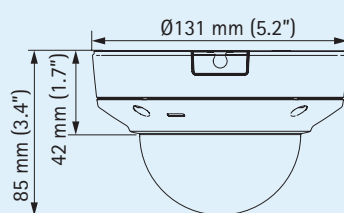
AXIS M3006-V
