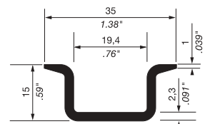
In compliance with EN 50022 standard (NFC 63015) DIN 3
